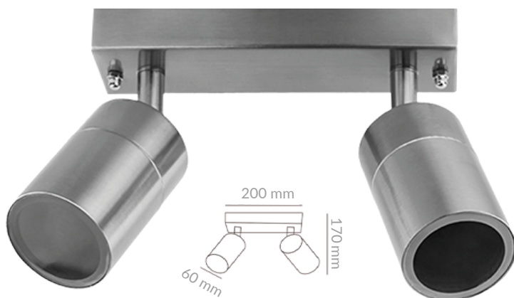
SMB-126A1
