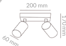
SMB-126A1
