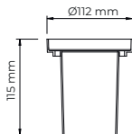
K008 Cánope IL60 Mark S & L
