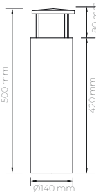
Dux poste de aluminio
