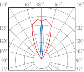
Óptica elíptica 14x34°
